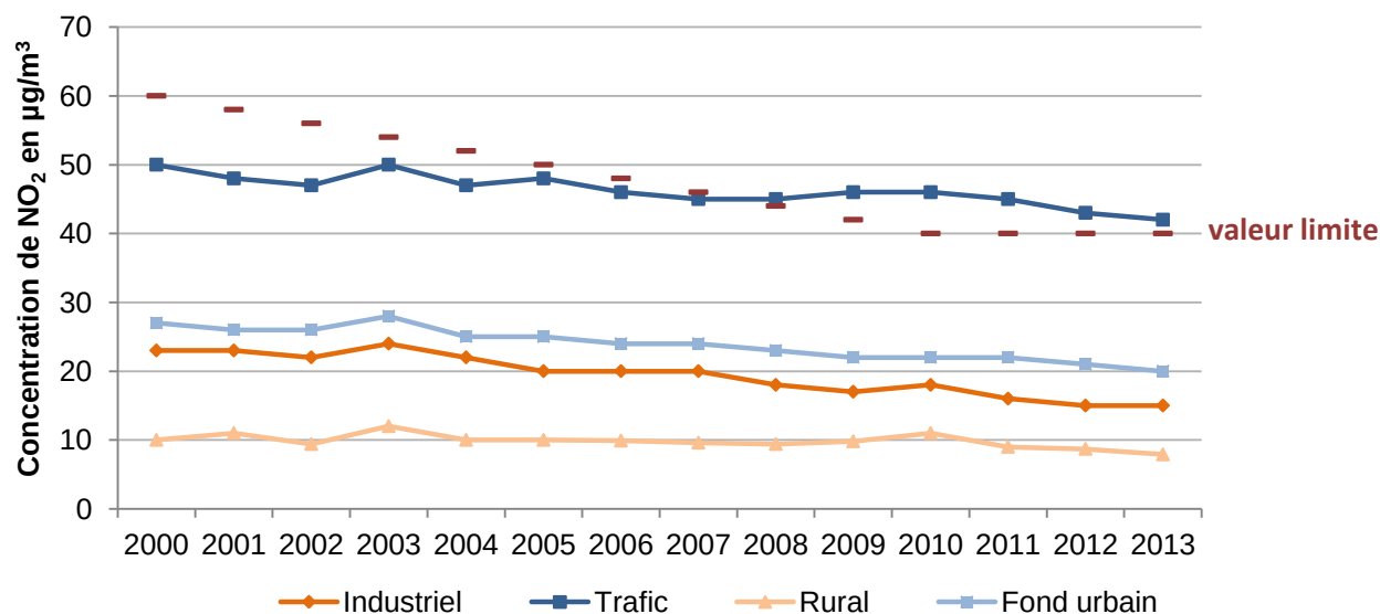
Graphique 1 : Évolution des concentrations moyennes annuelles en dioxyde d'azote (NO 2 ) entre 2000 et 2012 selon le type de site de mesure
